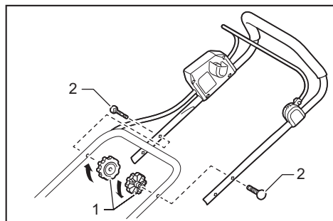
► 1. Tuerca de apriete 2. Tornillo de apriete
