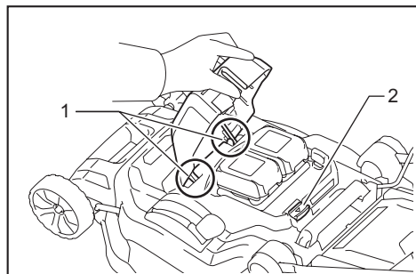
► 1. Punto de pivote 2. Palanca de bloqueo de la tapa de la batería
