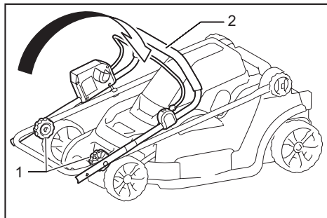
► 1. Tuerca de apriete 2. Asidero superior
