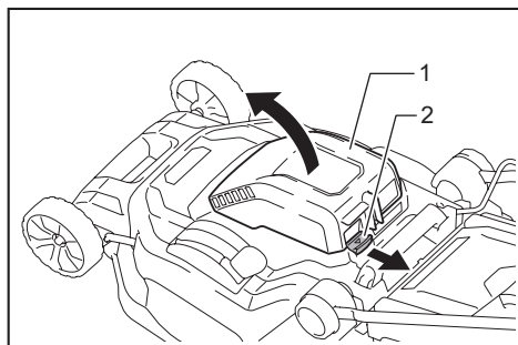
► 1. Tapa de la batería 2. Palanca de bloqueo de la tapa de la batería
