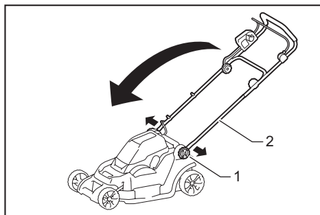
► 1. Tornillo de apriete 2. Asidero inferior
