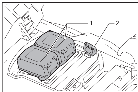
► 1. Cartucho de batería 2. Llave de bloqueo
