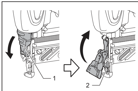
► 1. Latch 2. Door
