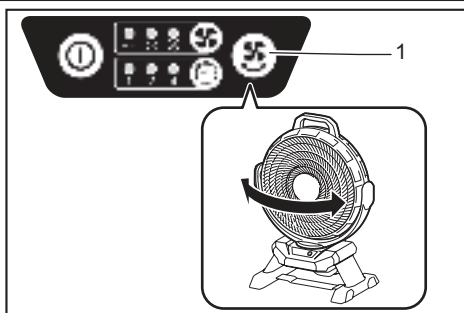
➤ 1. Bouton d'oscillation
