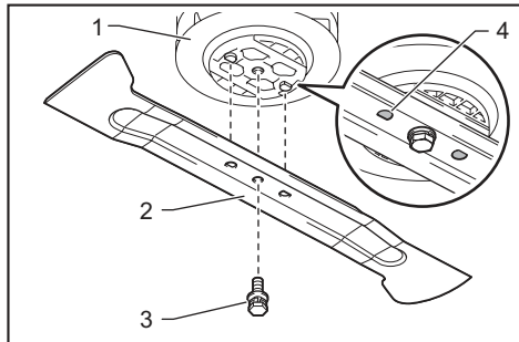
► 1. Soporte de la cuchilla 2. Cuchilla de cortacésped 3. Perno 4. Saliente
