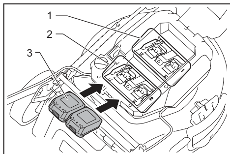
► (1) Puerto de batería 1 (2) Puerto de batería 2 (3) Cartucho de batería
