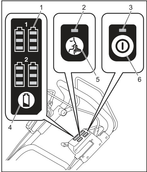
► 1. Indicador de batería 2. Lámpara de cambio de modo 3. Lámpara de alimentación principal 4. Botón de comprobación 5. Botón de cambio de modo 6. Interruptor de alimentación principal
