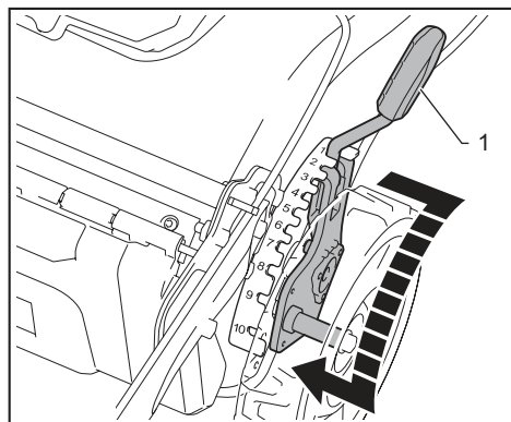
► 1. Palanca de ajuste de la altura de siega
