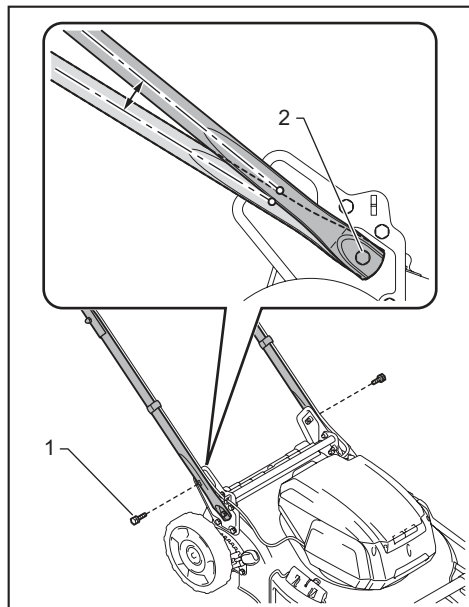
► 1. Perno superior 2. Perno inferior
