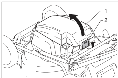
► 1. Tapa de la batería 2. Palanca de bloqueo
