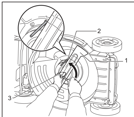
► 1. Cuchilla de cortacésped 2. Pasador 3. Llave de tubo
