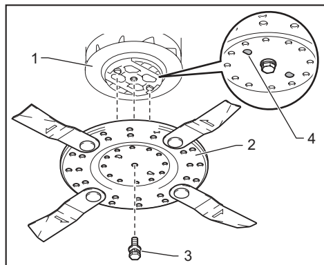
► 1. Soporte de la cuchilla 2. Placa de la base 3. Perno 4. Saliente
