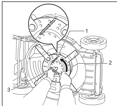
► 1. Pasador 2. Placa de la base 3. Llave de tubo
