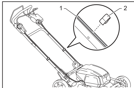
► 1. Cable 2. Soporte
