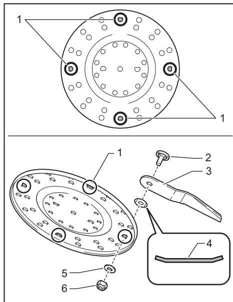
► 1. Orificio para perno 2. Perno 3. Cuchilla de cortacésped 4. Arandela de resorte 5. Arandela 6. Tuerca
