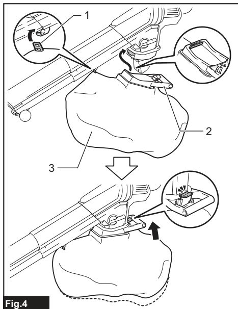
► 1. Claw 2. Handle 3. Dust bag
