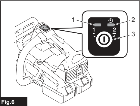
Fig. 6 ► 1. Lámpara de alimentación principal 2. Indicador de modo 3. Interruptor de alimentación principal
