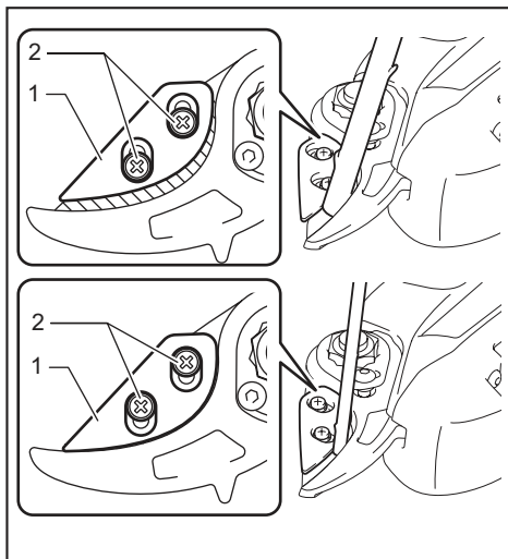
► 1. Agarrador 2. Tornillo
