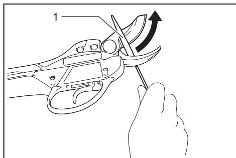
► 1. Lima adiamantada
