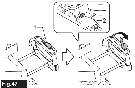
Fig.47 ► 1. Placa de apoio 2. Parafuso de aperto manual
