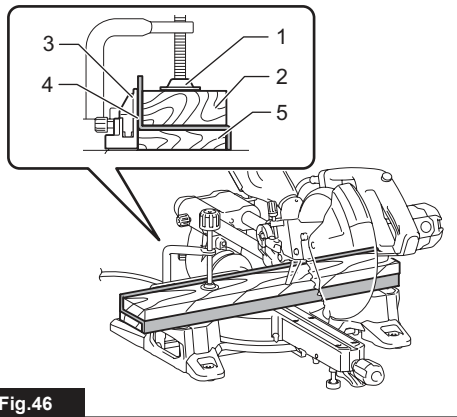
Fig.46 ► 1. Morsa 2. Bloco espaçador 3. Placa-guia 4. Extrusão de alumínio 5. Bloco espaçador
