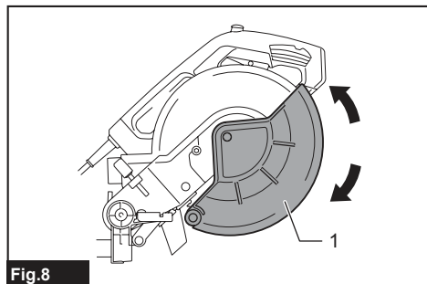
Fig. 8 ► 1. Protetor de segurança do disco
