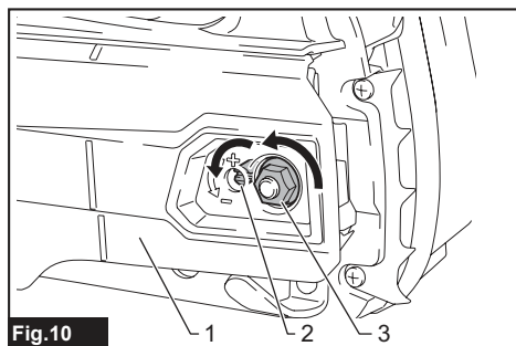
► 1. Cubierta del piñón 2. Tornillo de ajuste de la cadena 3. Tuerca de retención
