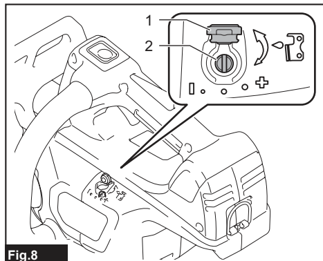
► 1. Tapón 2. Tornillo de ajuste
