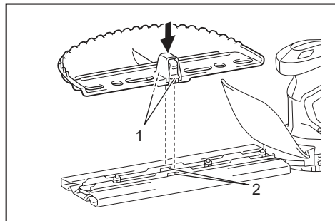
► 1. Ganchos 2. Agujeros
