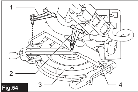
Fig. 54 ► 1. Tope de moldura corona izquierdo 2. Tope de moldura corona derecho 3. Base giratoria 4. Guía lateral
