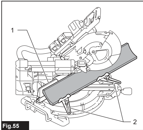
Fig.55 1. Guía lateral 2. Tope de moldura corona
