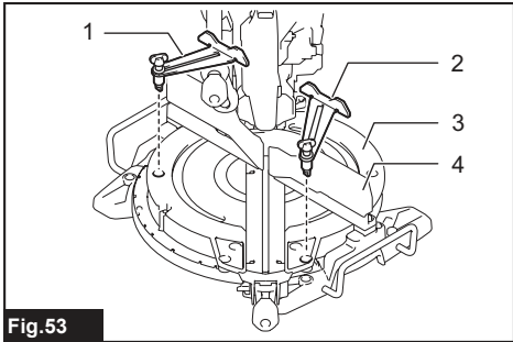
Fig. 53 ► 1. Tope de moldura corona izquierdo 2. Tope de moldura corona derecho 3. Base giratoria 4. Guía lateral
