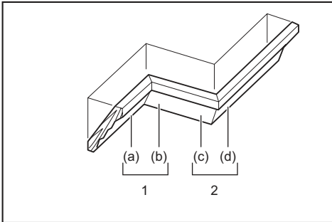
Fig.55 1. Guía lateral 2. Tope de moldura corona
