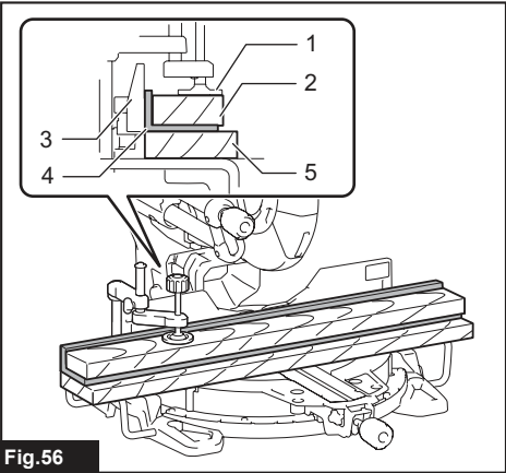
Fig.56 1. Mordaza 2. Bloque espaciador 3. Guía lateral 4. Extrusión de aluminio 5. Bloque espaciador
