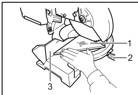
► 1. Escuadra 2. Mango 3. Guía lateral
