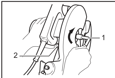
► 1. Llave de cubo 2. Bloqueo del eje
