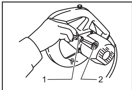
► 1. Atornillador 2. Tapa del portaescobillas
