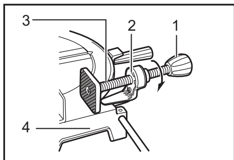
► 1. Pomo de la mordaza 2. Saliente 3. Eje de la mordaza 4. Base
