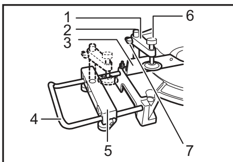
► 1. Brazo de la mordaza 2. Barra de la mordaza 3. Guía lateral 4. Soporte 5. Conjunto de soporte 6. Pomo de la mordaza 7. Tornillo
