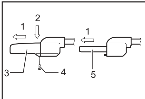
► 1. Extraer 2. Empujar 3. Caja de la lámpara 4. Tornillos 5. Tubo fluorescente
