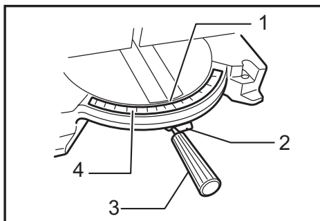
► 1. Flecha 2. Palanca de bloqueo 3. Mango 4. Escala de ángulo de inglete
