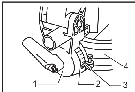
► 1. Brazo 2. Escala de bisel 3. Flecha 4. Base giratoria
