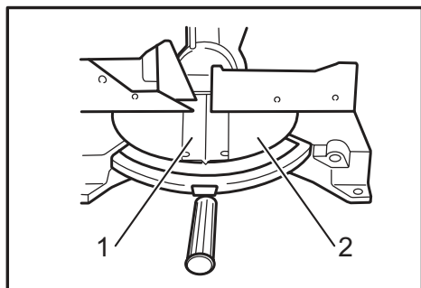
► 1. Placa de corte 2. Base giratoria
