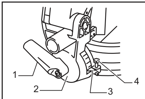
► 1. Palanca 2. Brazo 3. Flecha 4. Perno de ajuste del ángulo de bisel a 45°
