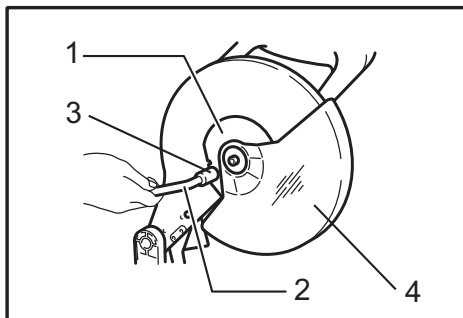
► 1. Cubierta central 2. Llave de cubo 3. Perno de cabeza hexagonal 4. Protector de disco
