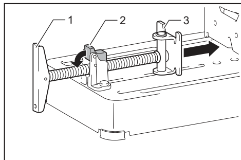
► 1. Mango 2. Soporte de rosca 3. Placa de mordaza 4. Placa de mordaza
