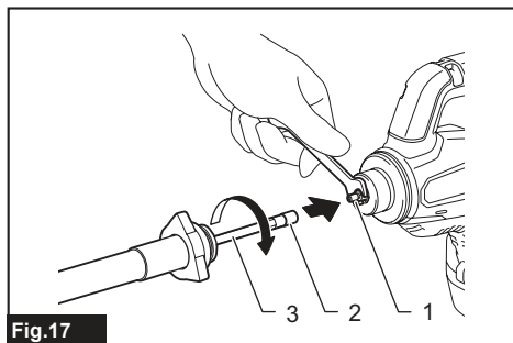
► 1. Eje motriz 2. Accesorio final 3. Eje tubular flexible
