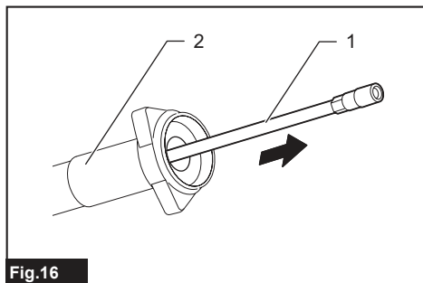
► 1. Eje tubular flexible 2. Envoltura exterior
