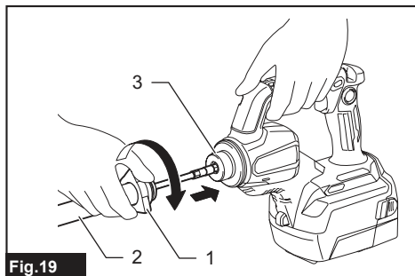
► 1. Acoplador 2. Envoltura exterior 3. Rosca exterior
